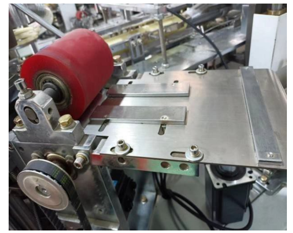
Altan Kağıt Besleme
