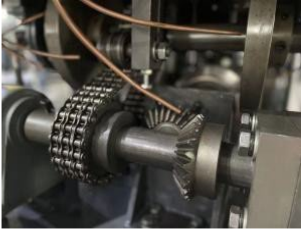
Üç Plakalı Zincir ve Dişliler
