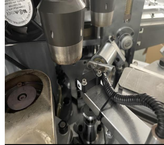
SENSÖR 1, ÜST NAMLUYU ALGILAR
