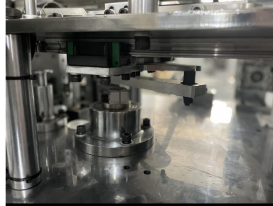
KAĞIT ÇEKME MEKANİZMASI
